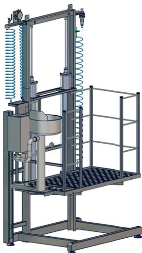
Plošina pneumatická / Площадка пневматическая / Pneumatic platform / pneumatische Plattform
